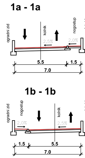
POPREČNI PRESJCI MJ 1:250
